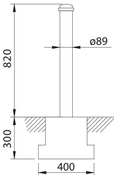
Trafik stele stationær- her vist støbt 180 mm ned i betonfod
