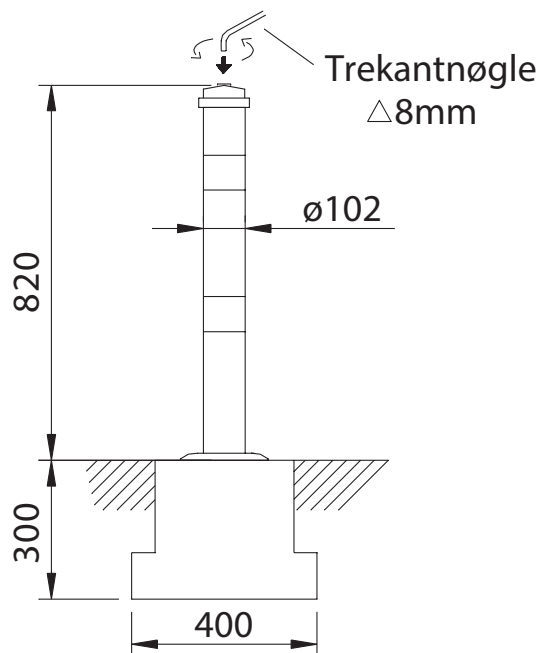
Trafik stele flytbar - her vist med betonfod og indstøbt stålplade til fastgørelse af stele
