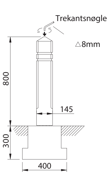
Park steele flytbar vist med betonfod og indstøbt stålplade til fastgørelse af steele
