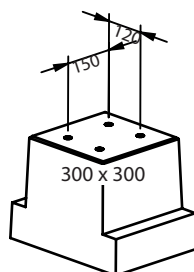
Præfabrikeret beton fundament til den stationære og nedfældbare Park-Click
