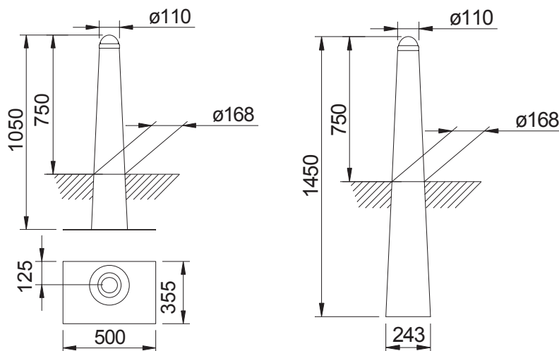
Amsterdam fjedrende stele med stålplade til støbning i beton
